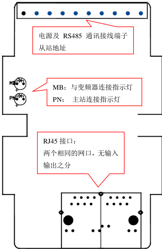
图 3 PNTOMM外置模块布局图
