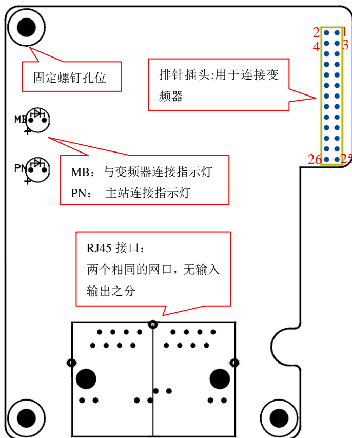
图 2 PNTOMM 内插卡布局图
