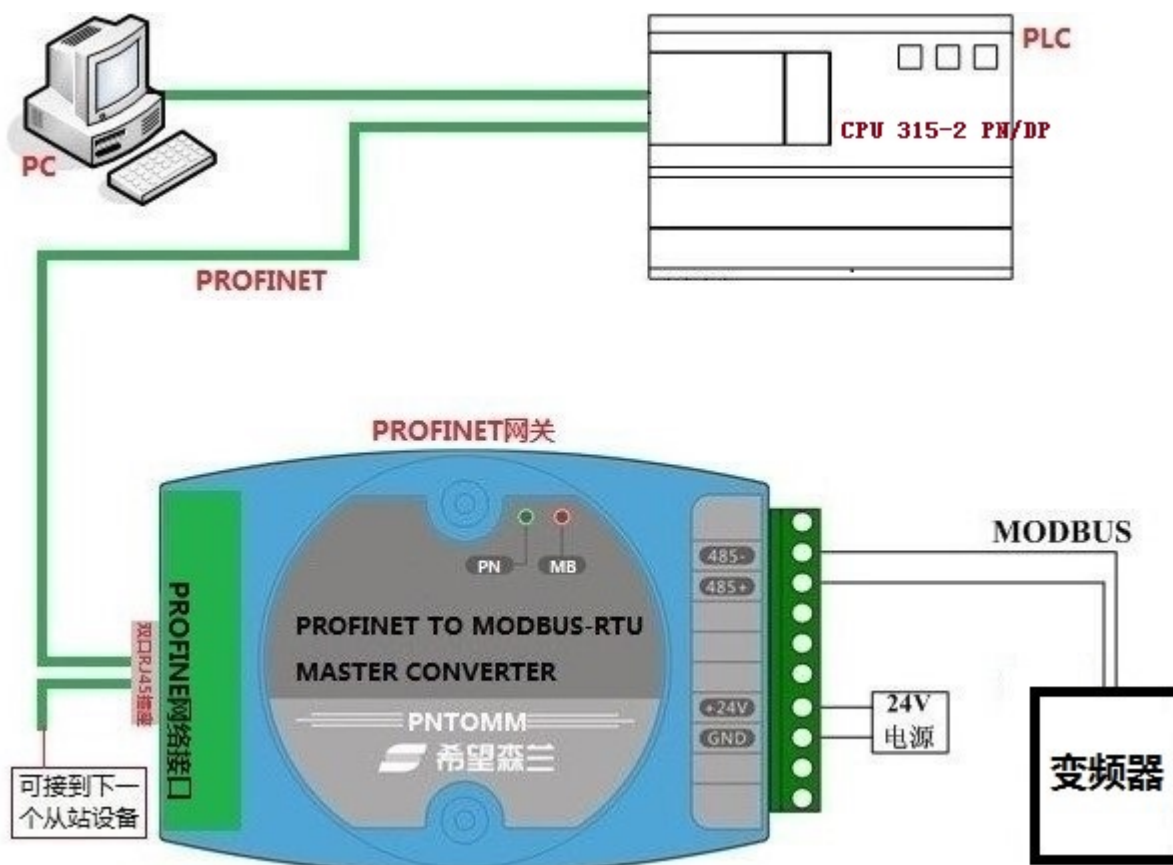
图 5 硬件接线示意图
