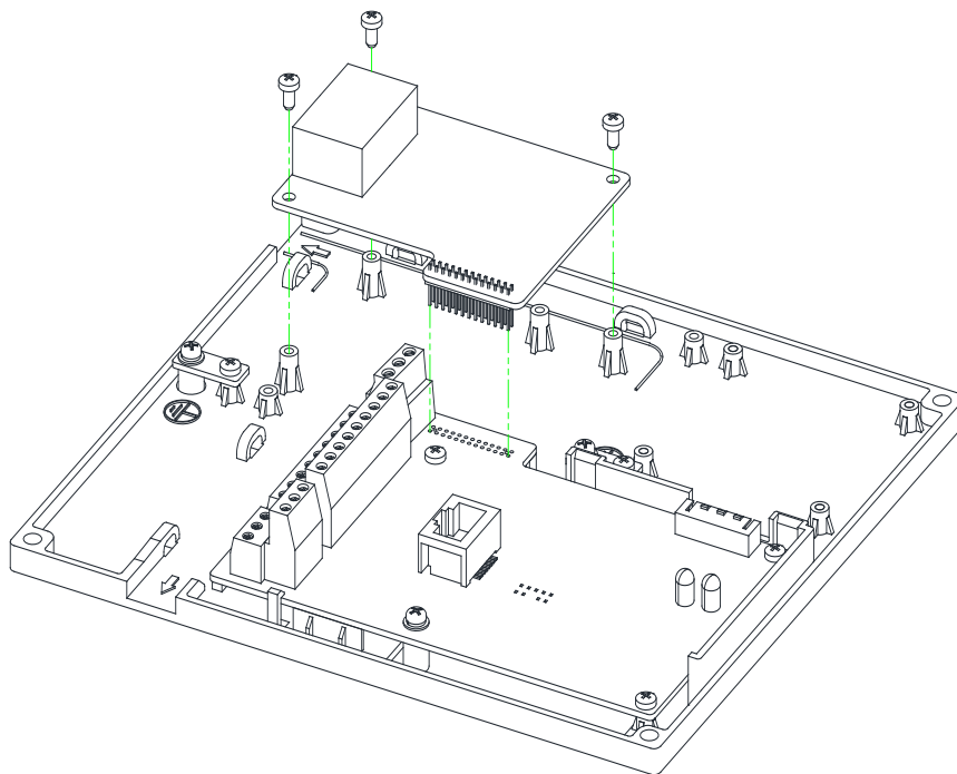
图 1 PNTOMM 内插卡安装示意图
